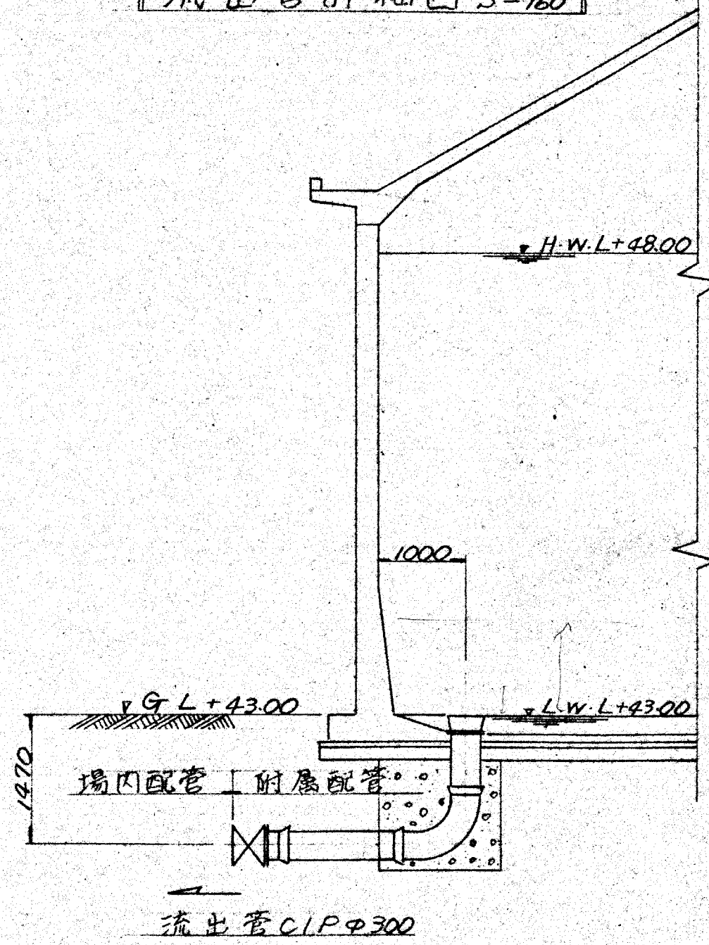
流出管詳細図 S=1/60
