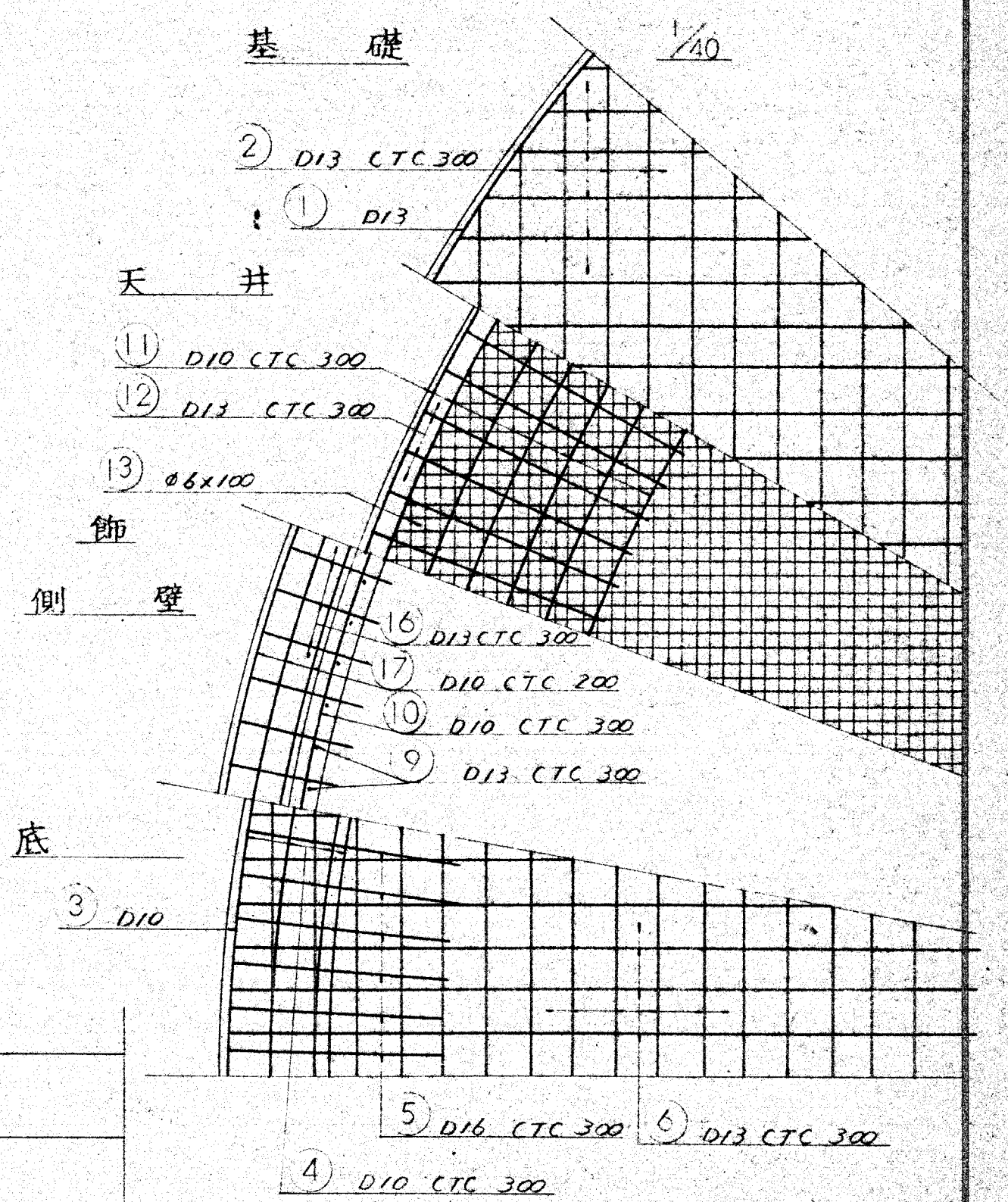
平面図
