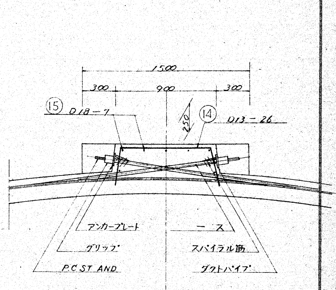
定着部
