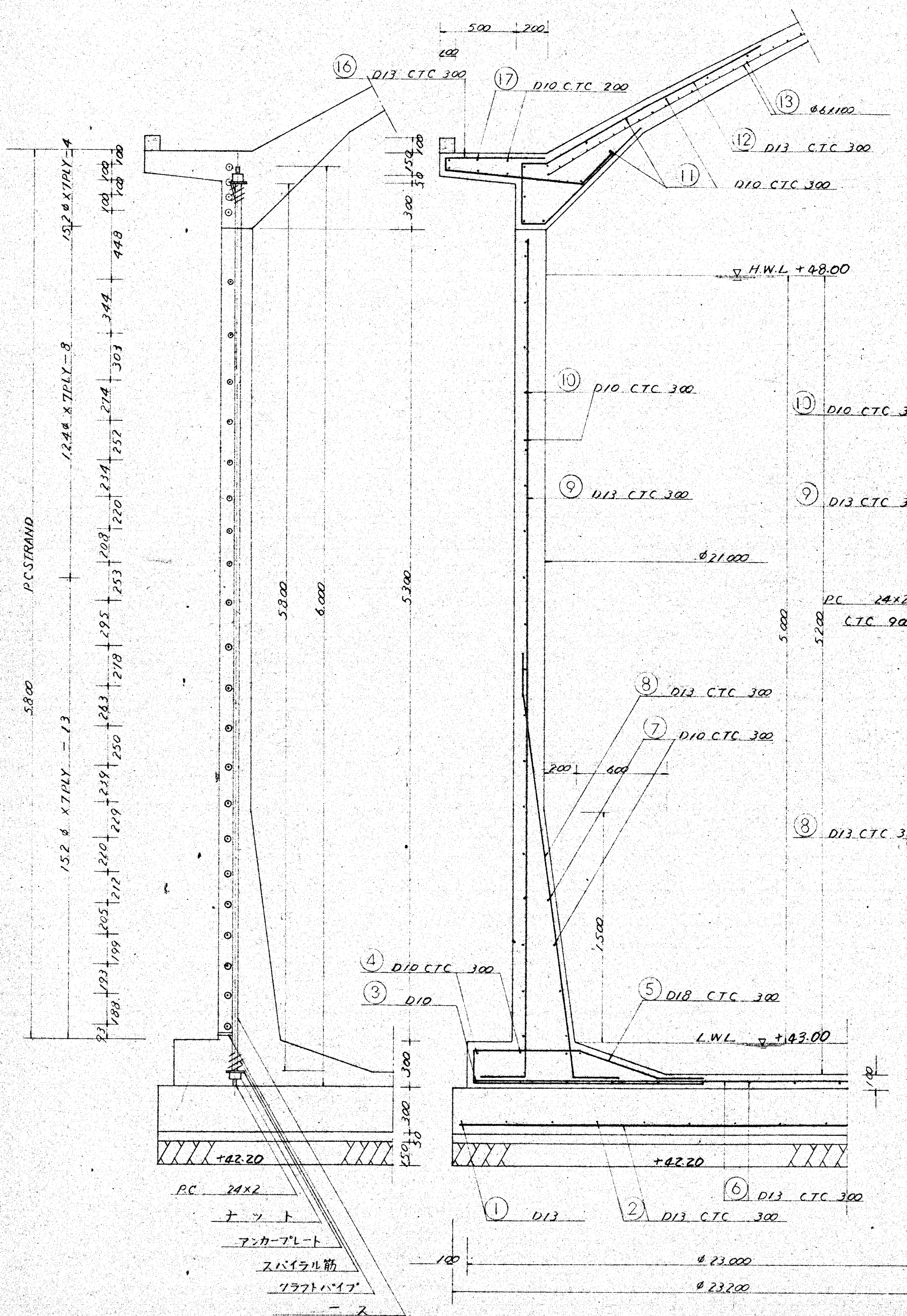
PC材配置図
