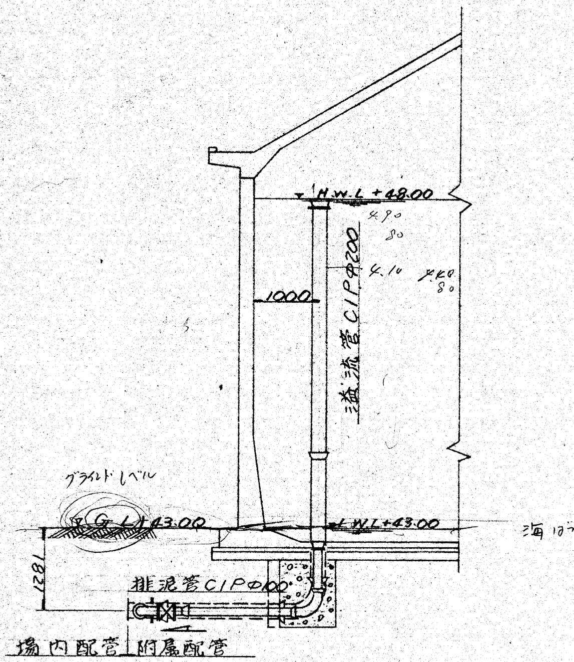
排泥溢流管詳細図 S=1/60
