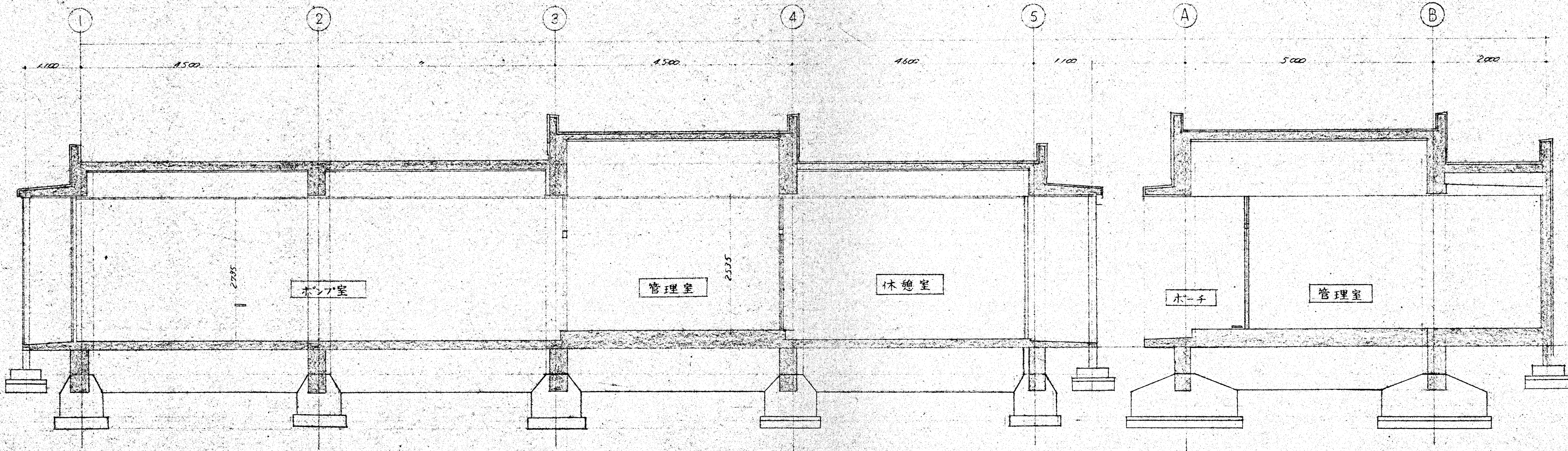
断面図 1/50
