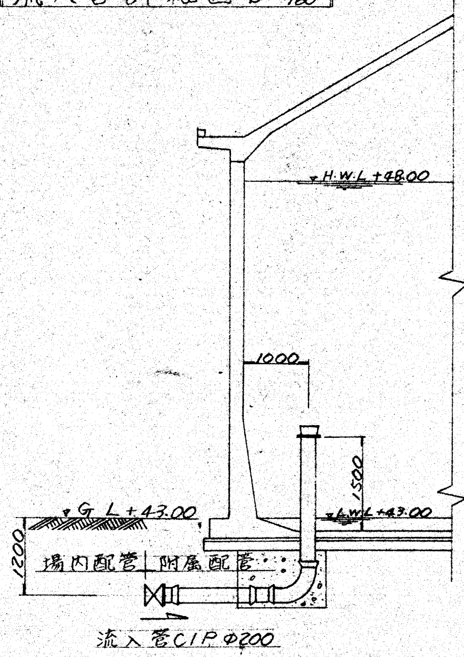
流入管詳細図 S=1/60
