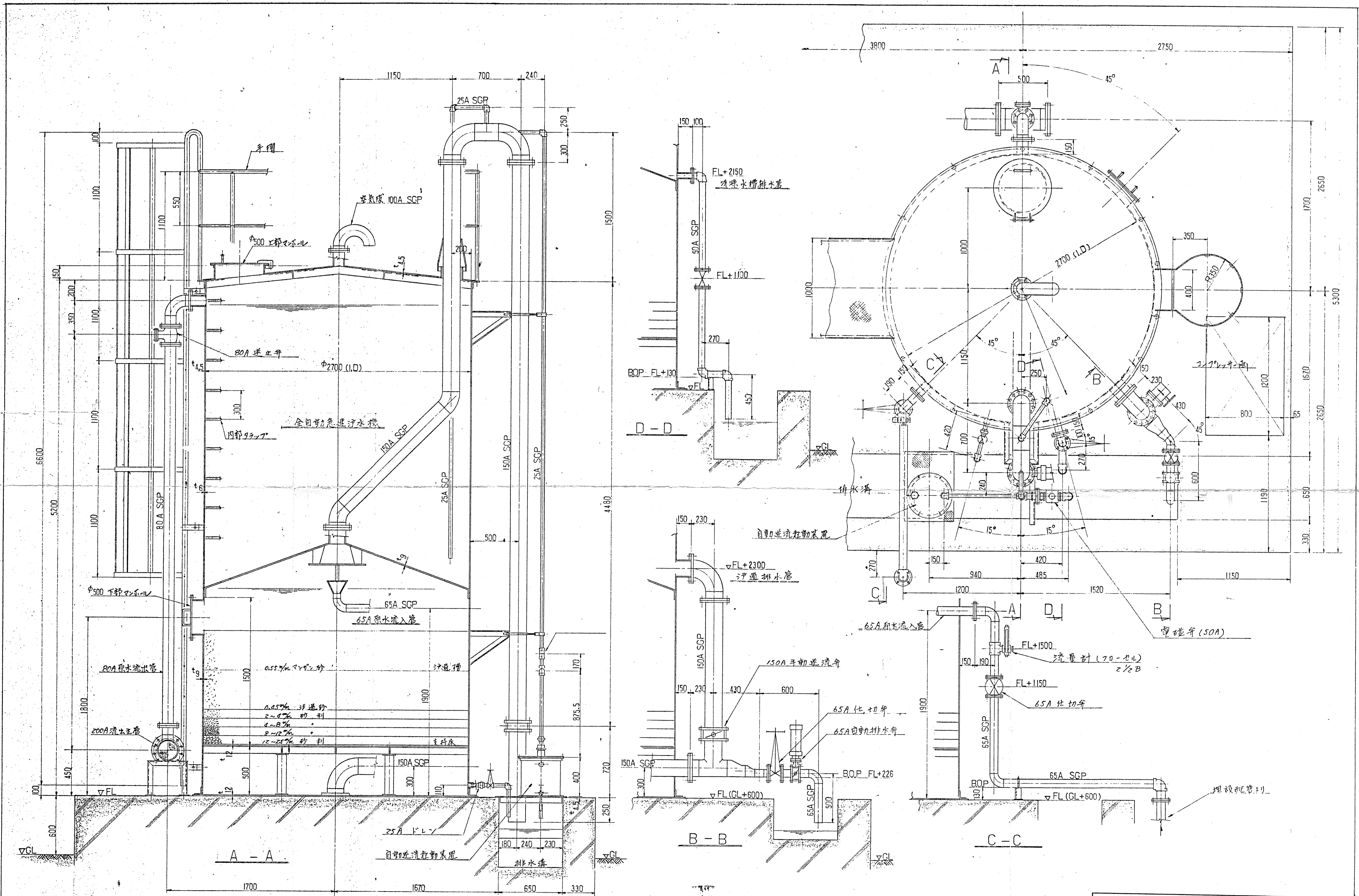
川西町水道事業変更認可設計図 図名 急造ろ過機構造図 縮尺 1/20 図番 8/27 磯城郡川西町
