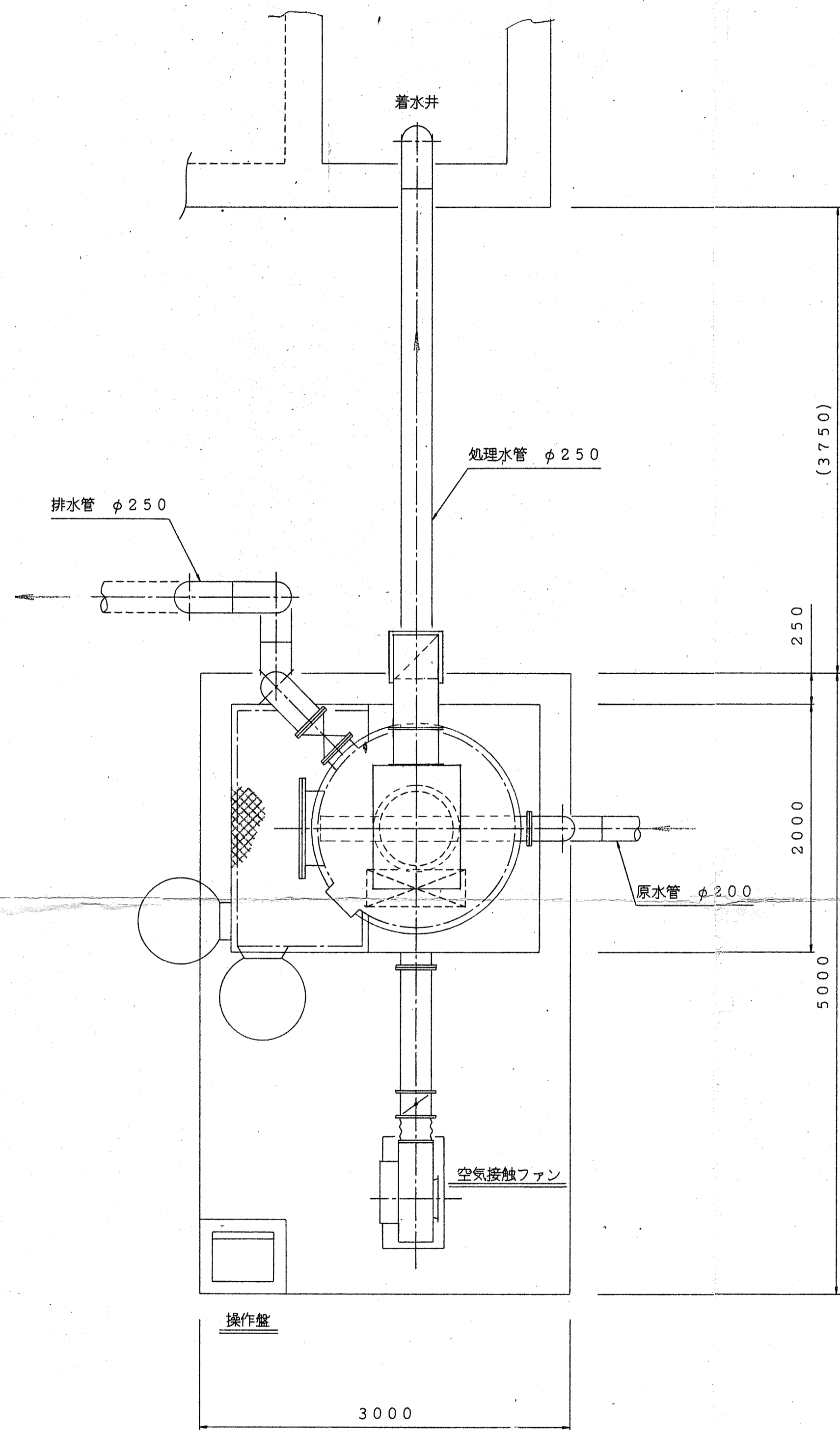
平面図 (S=1/30)
