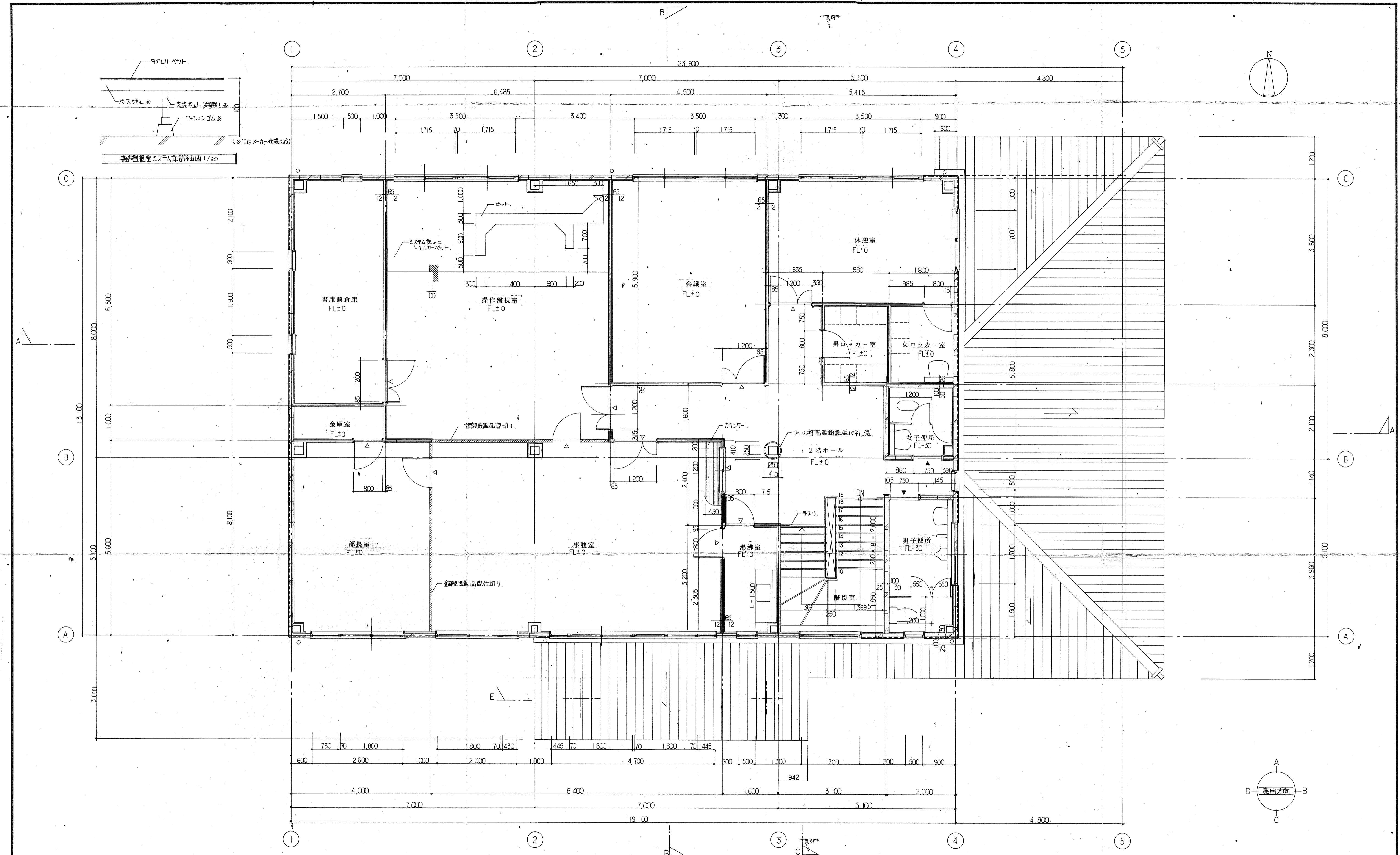
2F 平面詳細図 S=1:50
