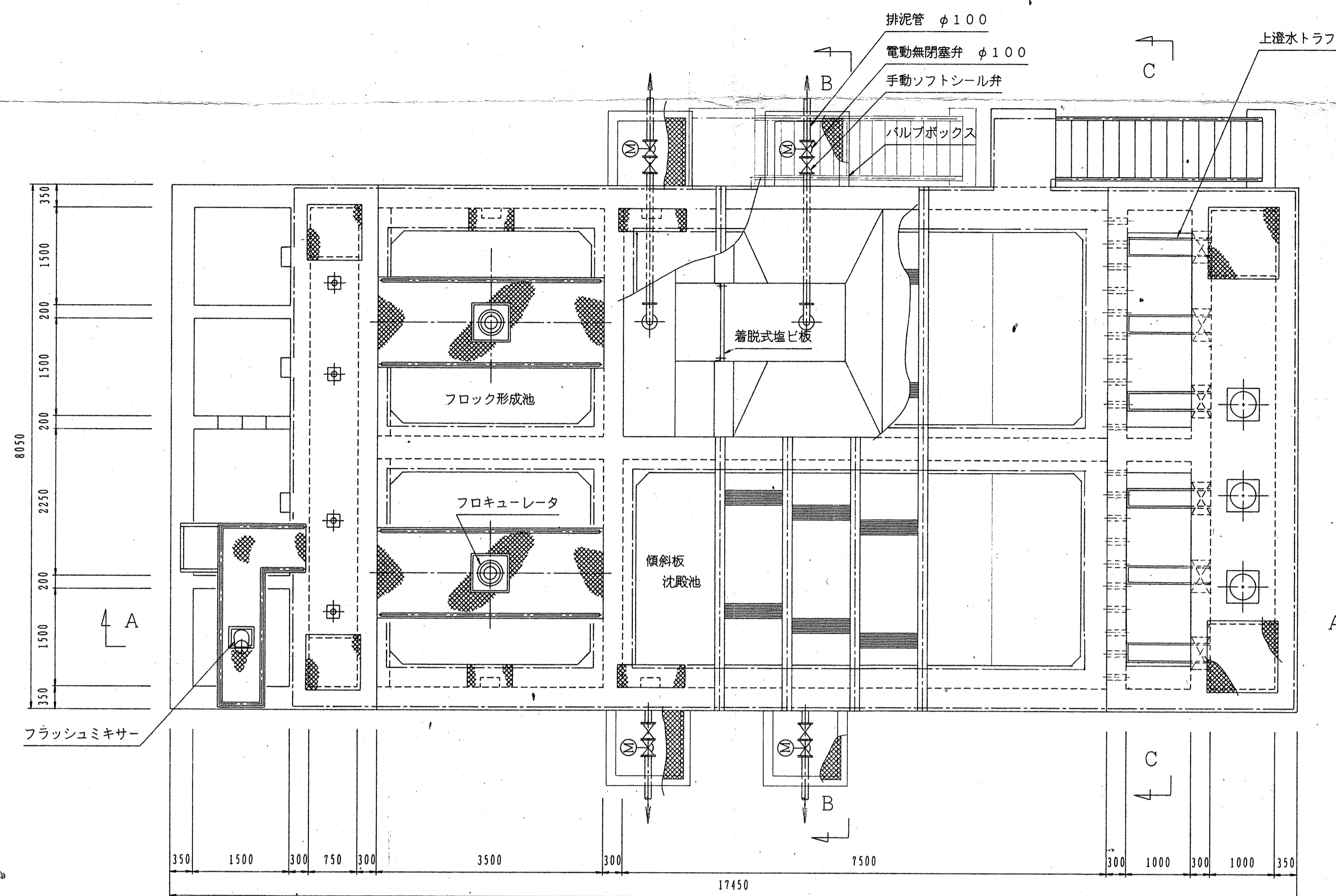
平面図 (S=1/50)
