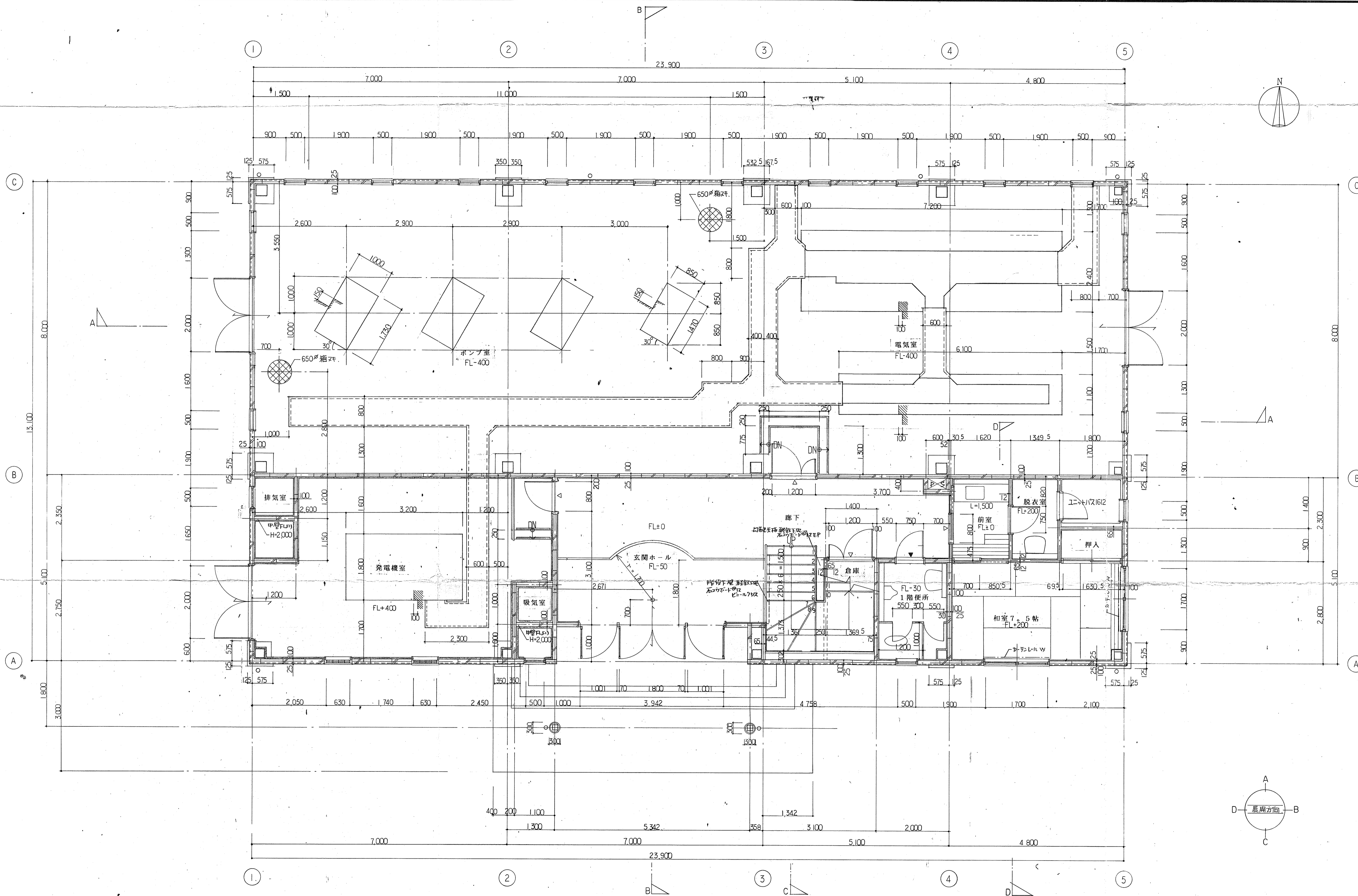
1F 平面詳細図 縮尺 1:50
