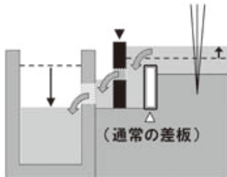
田んぼダムを実施した場合
