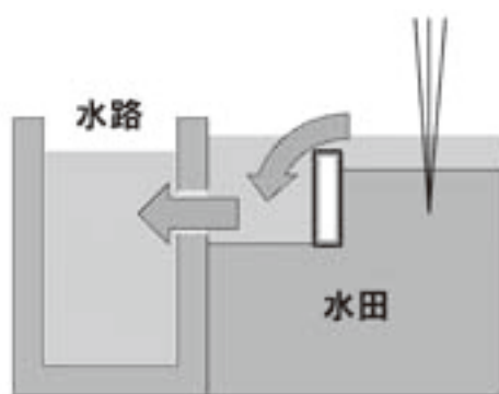
田んぼダムを実施していない場合
