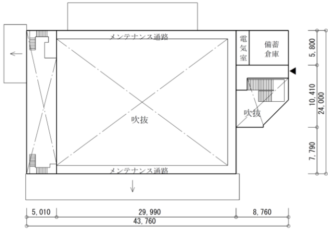
屋内運動場 2階平面図
